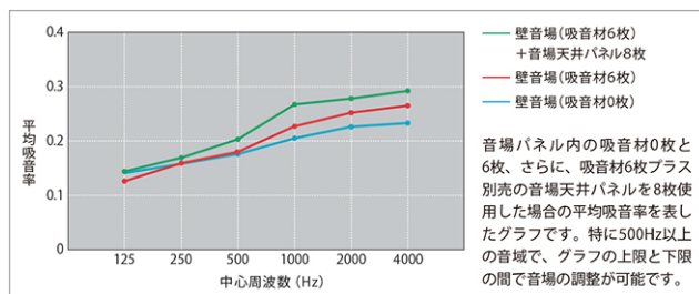
平均吸音率の調整可能範囲(3.0畳タイプ)
