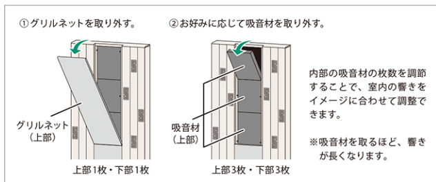
好みの響きに調整できる音場壁パネル
