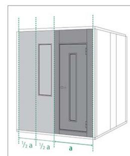
統一化された規格サイズ
