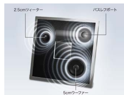
2ウェイ構成のスピーカーユニット
